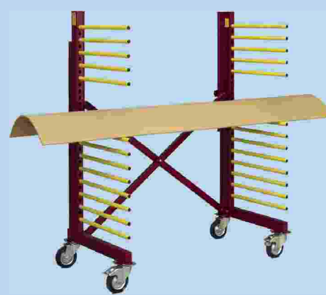
Gedemonteerde armen bij een R660-X
